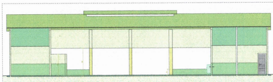
CORTE 4 ESCALA - 1:50
