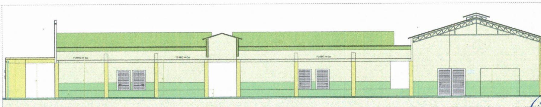
CORTE 6 ESCALA - 1:40
