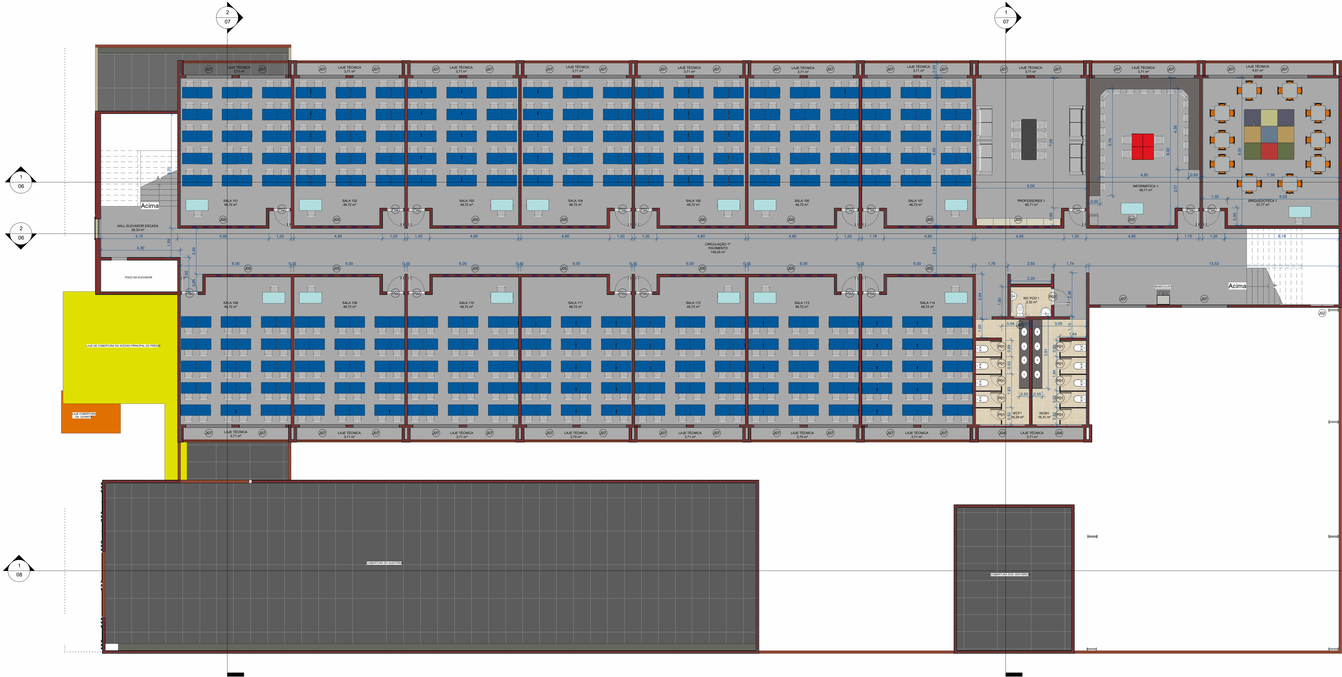
1 PLANTA BAIXA - 1º PAV 1 : 100
