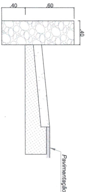
Detalhes De Parede de contenção e Sarjeta
