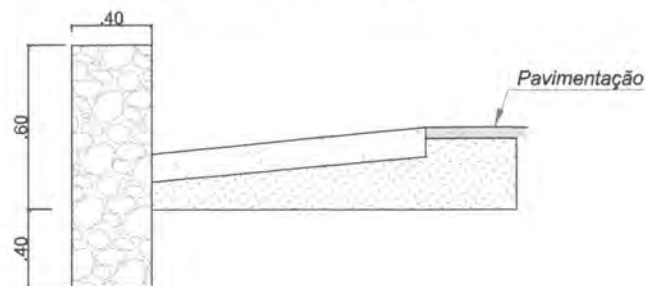
Detalhes De Parede de contenção e Sarjeta
