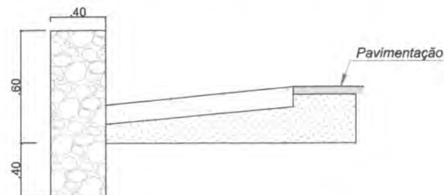
Detalhes De Parede de contenção e Sarjeta
