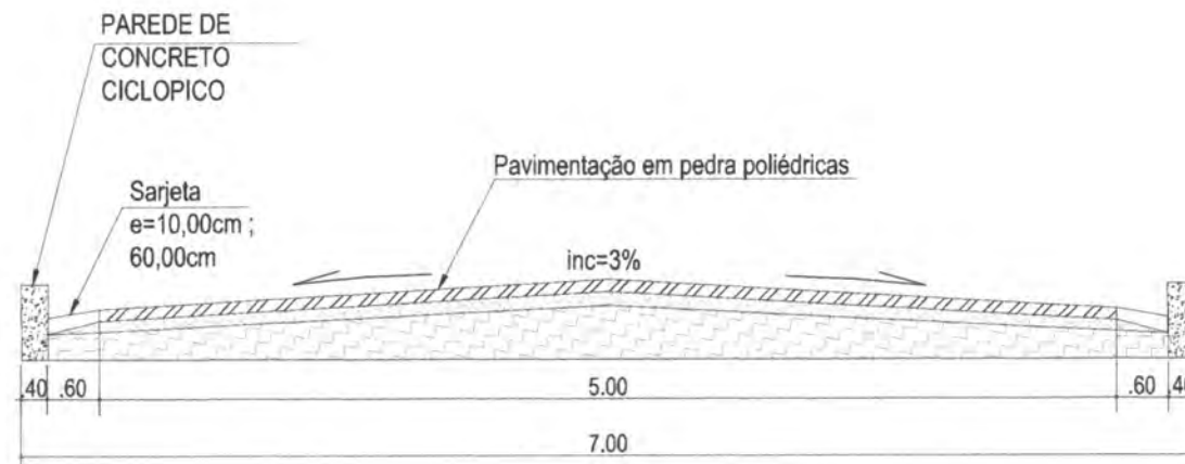
Detalhes De Parede de contenção e Sarjeta
