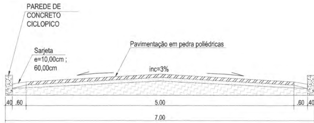
Detalhes De Parede de contenção e Sarjeta
