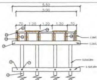
ESQUEMA LONGITUDINAL ESCALA 1:50
