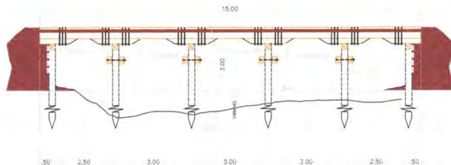
ESQUEMA LONGITUDINAL ESCALA 1:50
