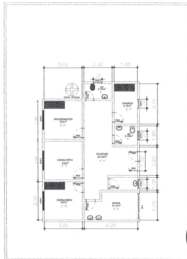
PLANTA DEMOLIR/CONSTRUIR esc 1:50
