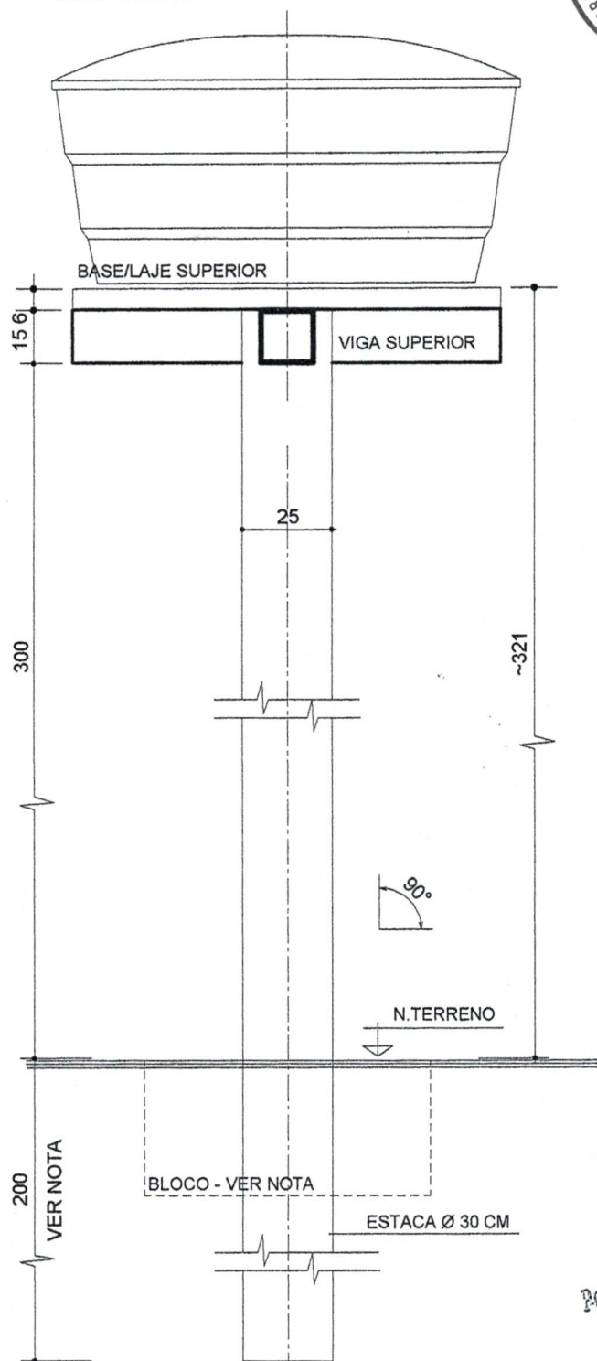
DETALHE - TORRE DE ELEVAÇÃO - TIPO 01
