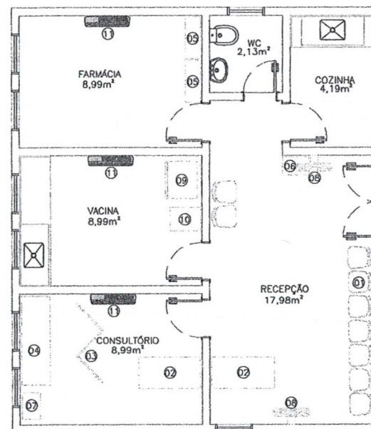
PLANTA MOBILIADA
