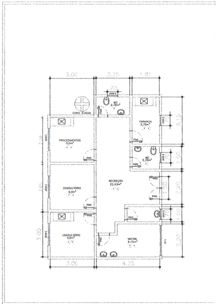
PLANTA BAIXA ATUAL esc 1:50
