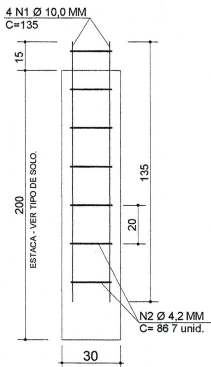
ESTACA
