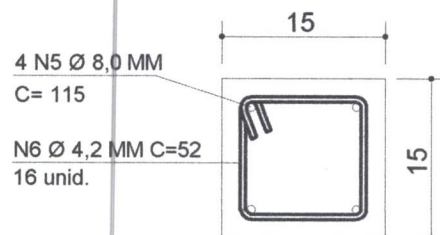
CORTE BB - VIGA/SUPERIOR
