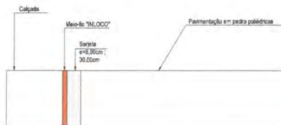
DETALHE DA PAVIMENTAÇÃO
