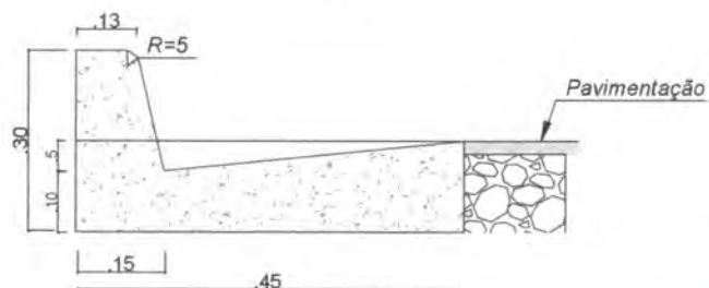
Detalhes do Meio Fio e Sarjeta
