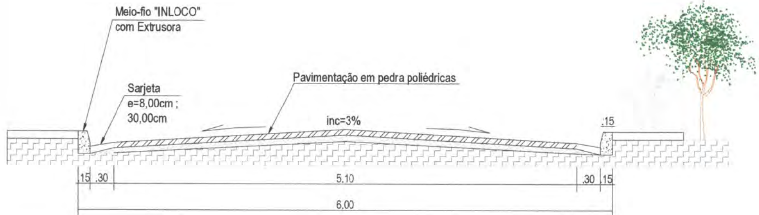
Detalhes do Meio Fio e Sarjeta
