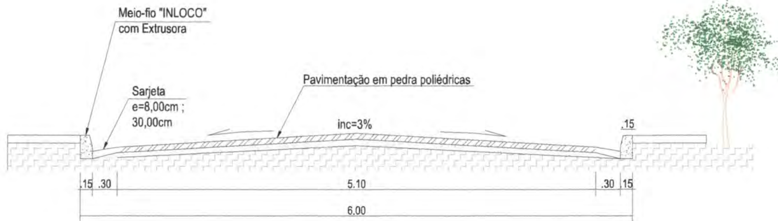
Detalhes do Meio Fio e Sarjeta
