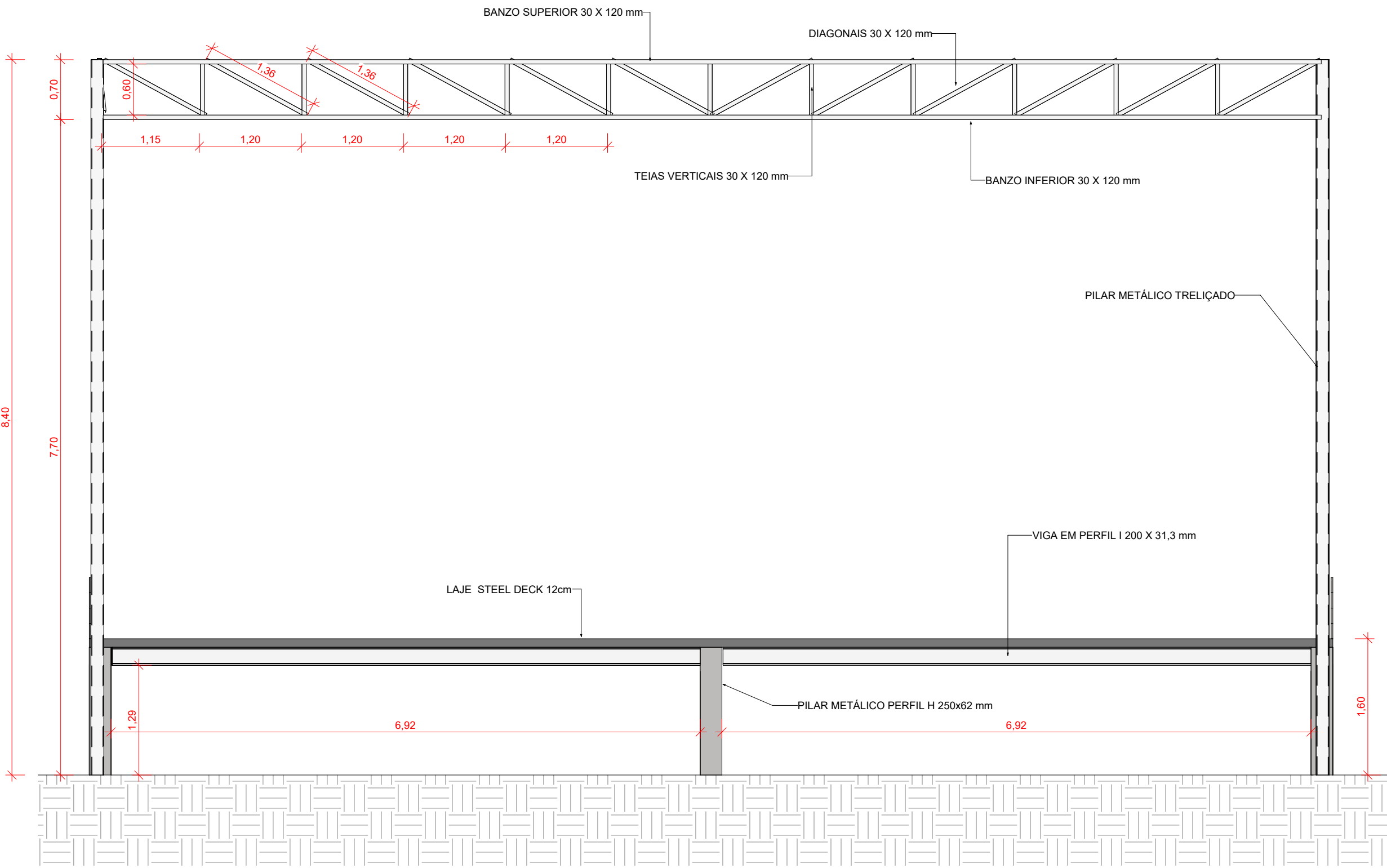
1 VISTA FRONTAL - ESTRUTURA METÁLICA
