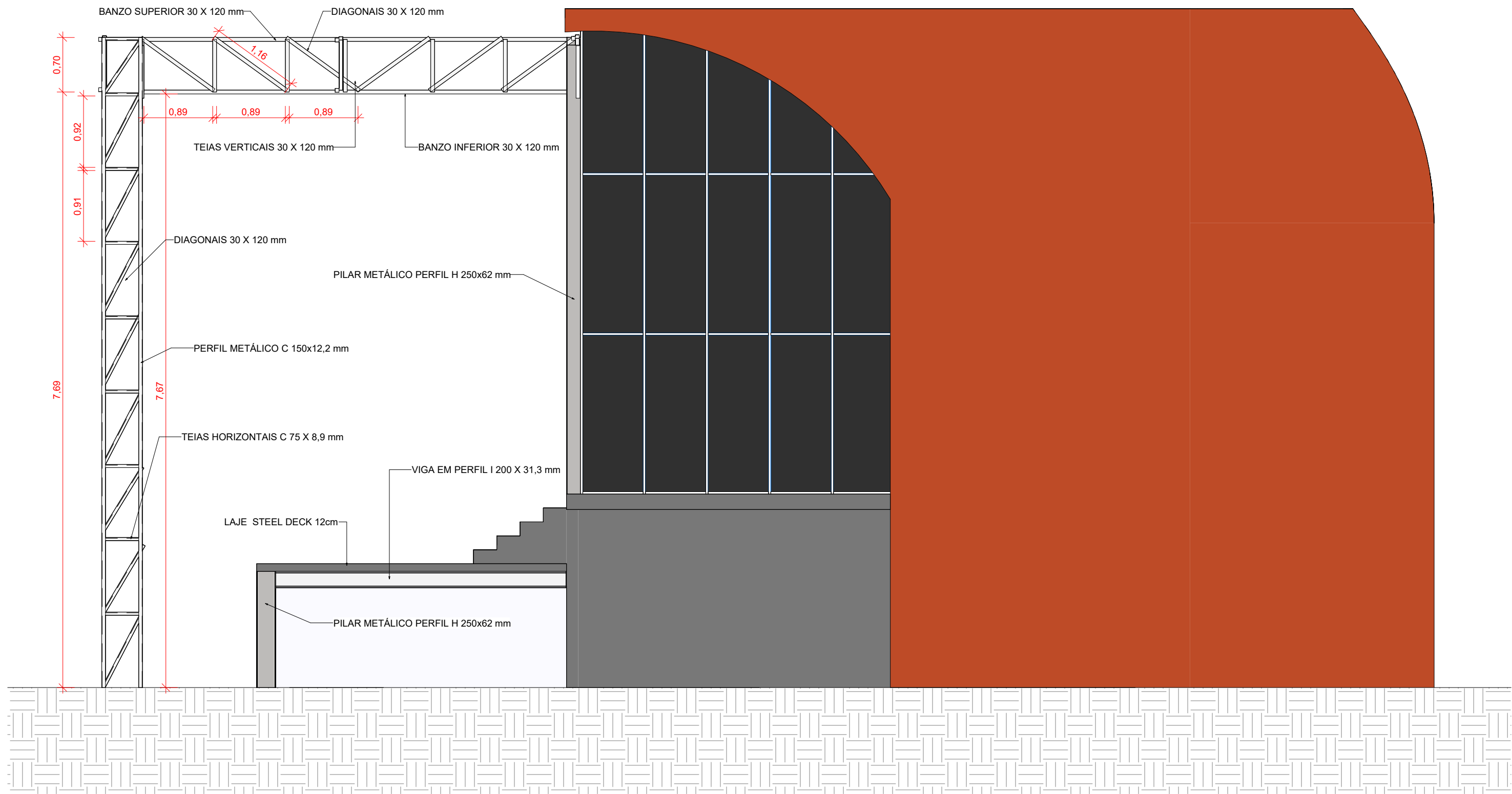
2 VISTA LATERAL - ESTRUTURA METÁLICA
