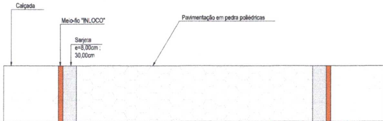
DETALHE DA PAVIMENTAÇÃO
