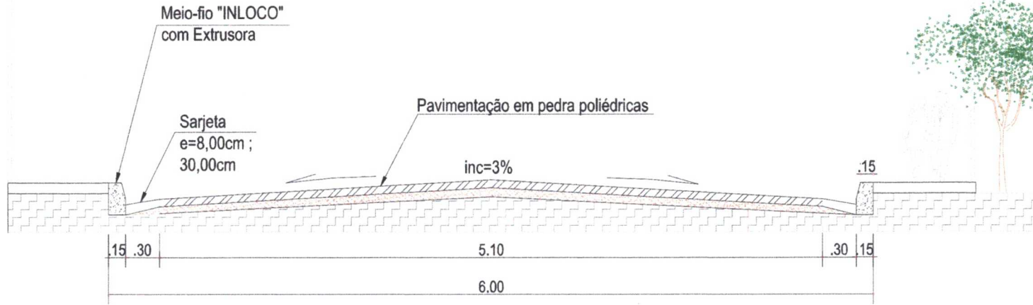
Detalhes do Meio Fio e Sarjeta
