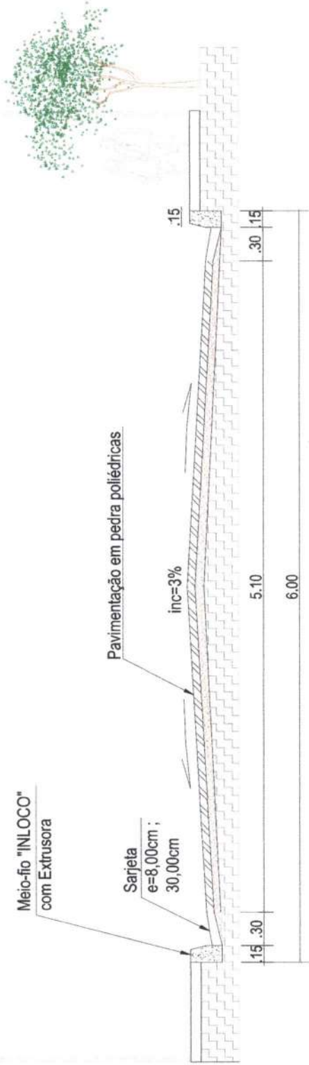
DETALHE DA PAVIMENTAÇÃO
