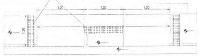
DETALHE DA ACESSIBILIDADE - SERÁ IMPLEMENTADAS RAMAS COM 113C TÁTIL EM CAÇADAS JÁ EXISTENTE
