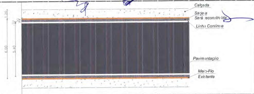
DETALHE DA PAVIMENTAÇÃO
