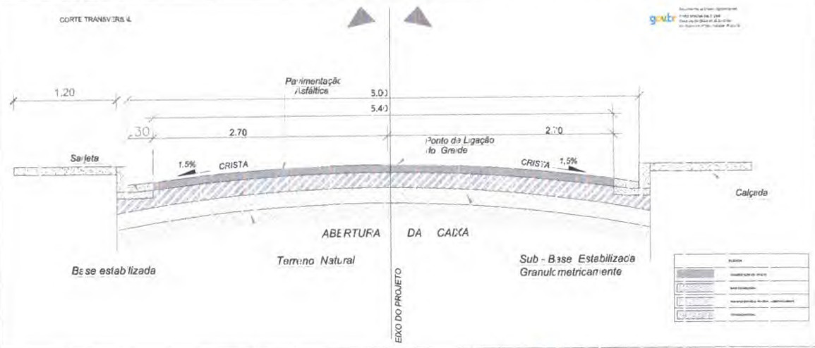
DETALHE DA PAVIMENTAÇÃO
